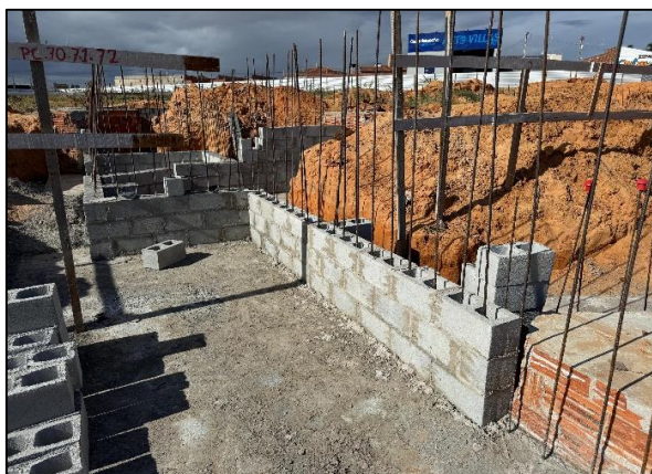
Foto 11: Execução de parede estrutural em etapa de contenção
