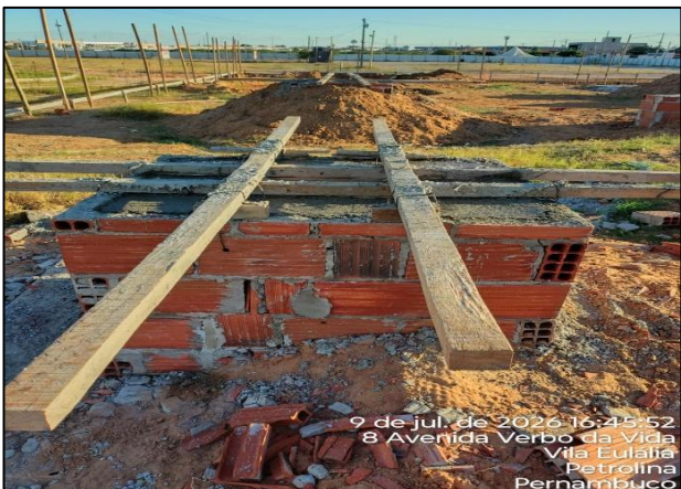
Foto 4: Execução de concretagem manual de cálice de sapata de fundação
