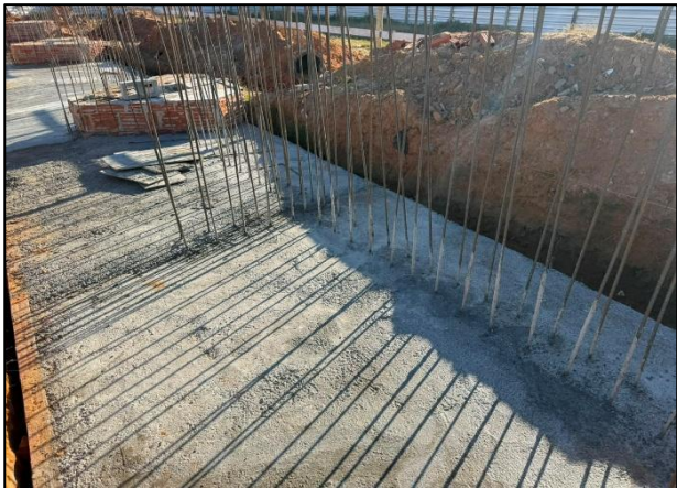
Foto 9: Execução de base para contenção (sapata corrida) 35cm de altura com 2,5m de largura.
